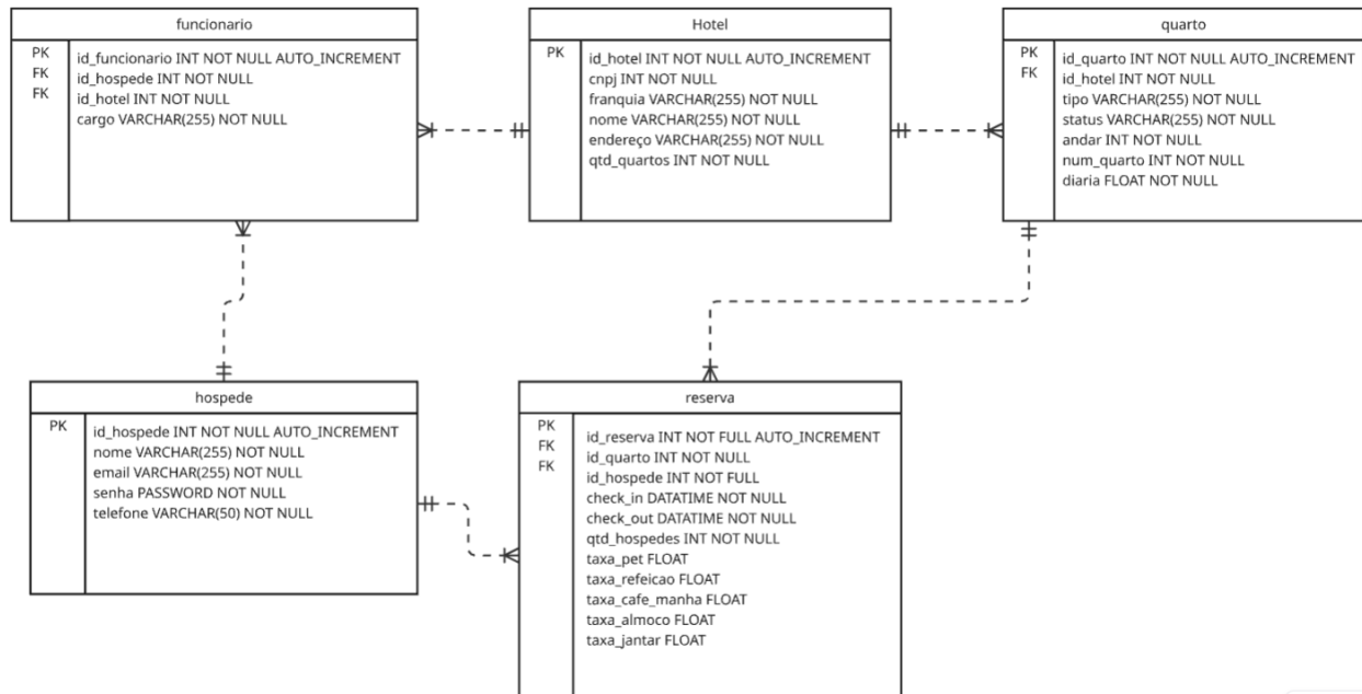
Figura 12 – Modelagem lógica do banco de dados do Anfitrião
