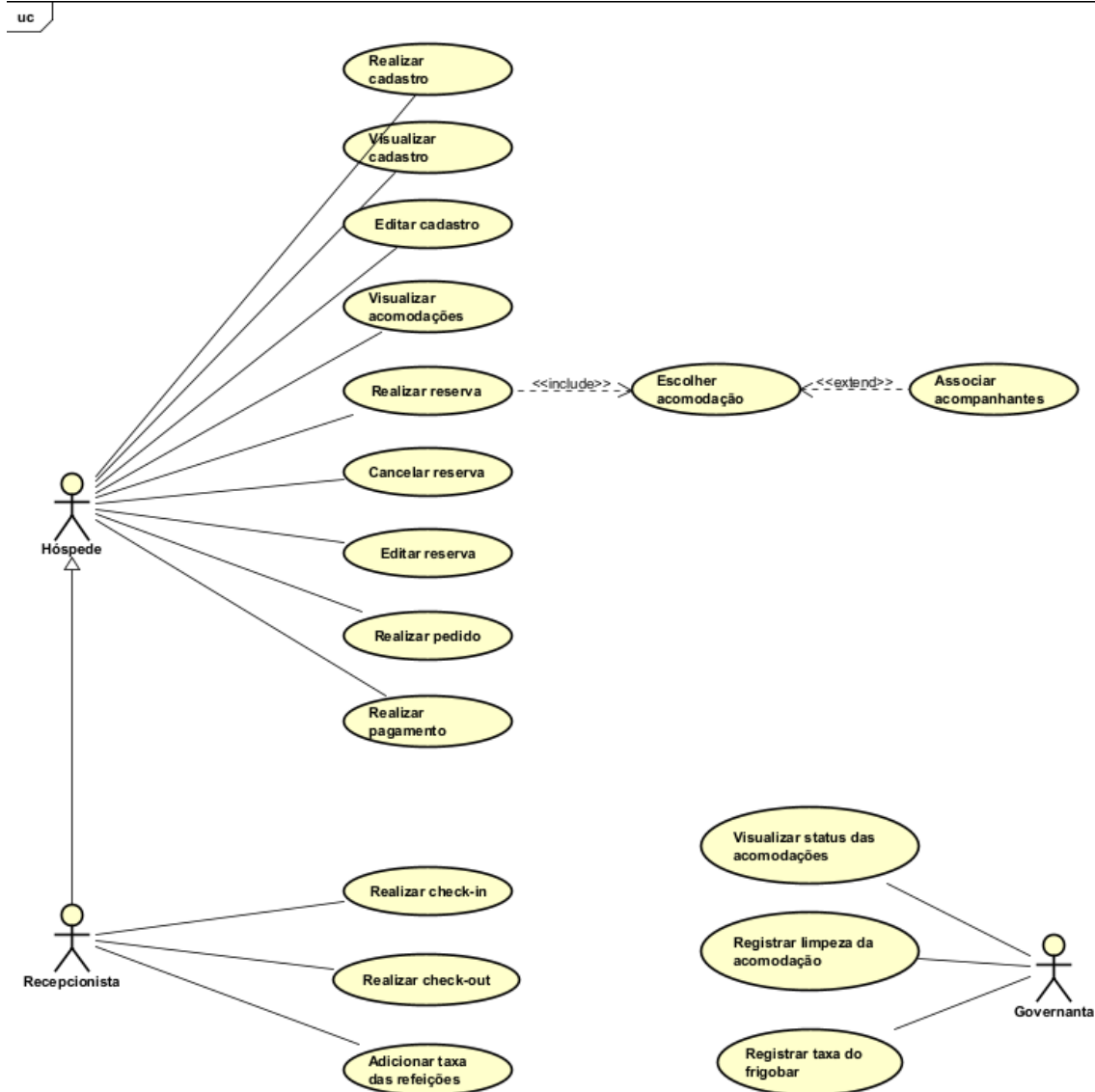
Figura 11 – Diagrama de caso de uso do Anfitrião
